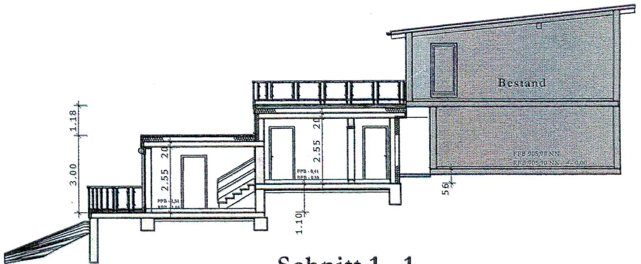
Schnitt 1 - 1
