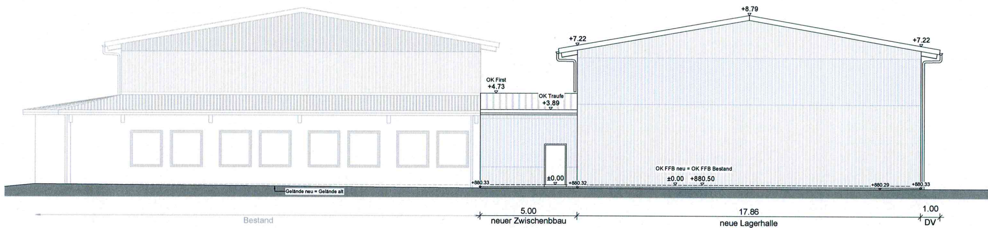
Ansicht Ost
