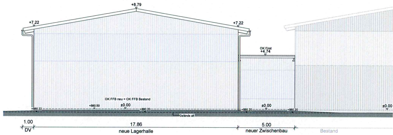
Ansicht West
