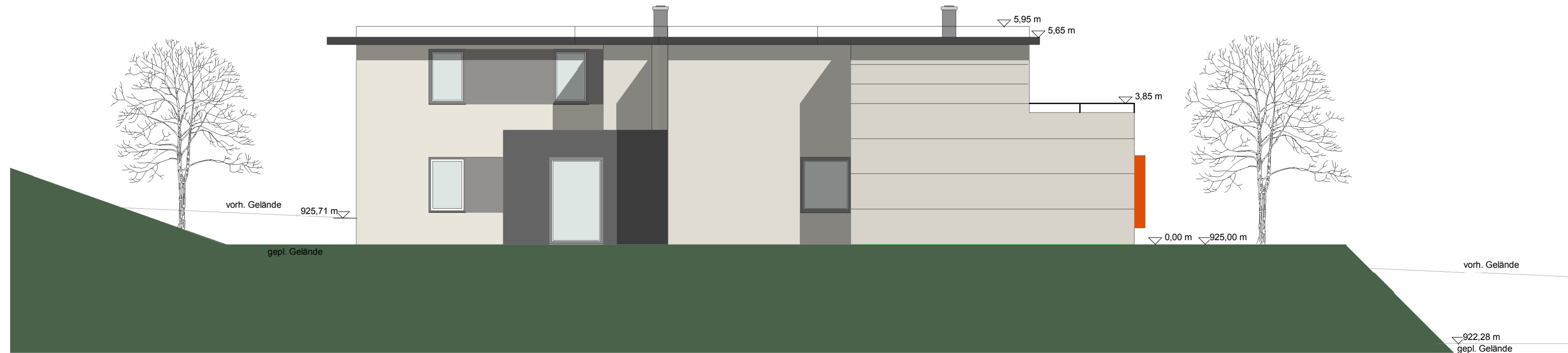
1 Ansicht Nord 1 : 100
